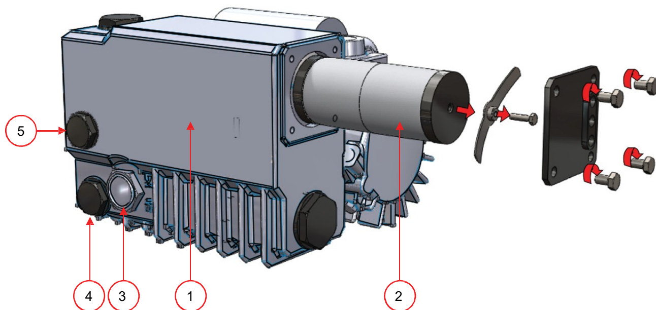
Rys. 3: PRZEGLĄD POMPY (Z USUNIĘTĄ OSŁONĄ)
