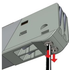
Rys. 12: Wymiana listwy zgrzewającej
